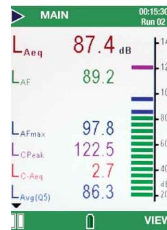
Breitbandmessung
