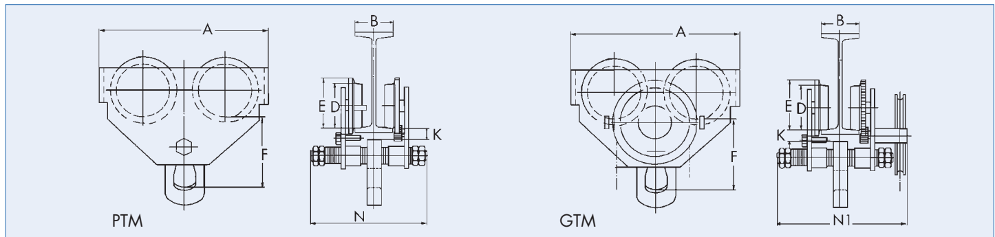
Haspelkettenlaufkatze GTM
