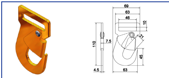
Art.-Nr. 92 Endbeschlag für Zurrleiste
