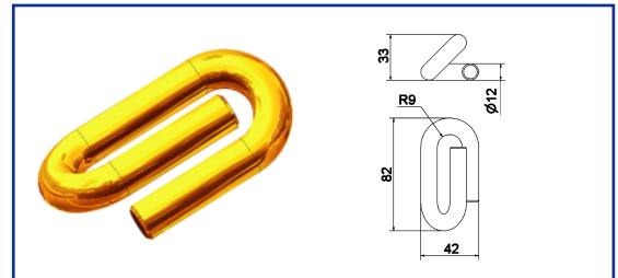
Art.-Nr. 80459 Agraffe
