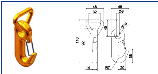
Art.-Nr. 4071 Karabinerhaken
