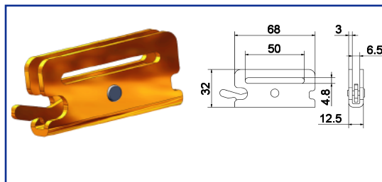
Art.-Nr. 92 Endbeschlag für Zurrleiste
