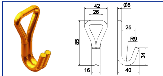
Art.-Nr. 2050 edrehter Karabinerhaken mit Triangel
